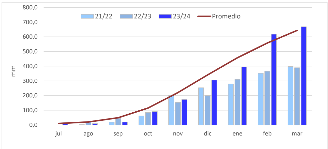
Gráfico 2: Registro del Total de precipitaciones durante el periodo cultivos de verano (línea marrón continua es el promedio histórico).
