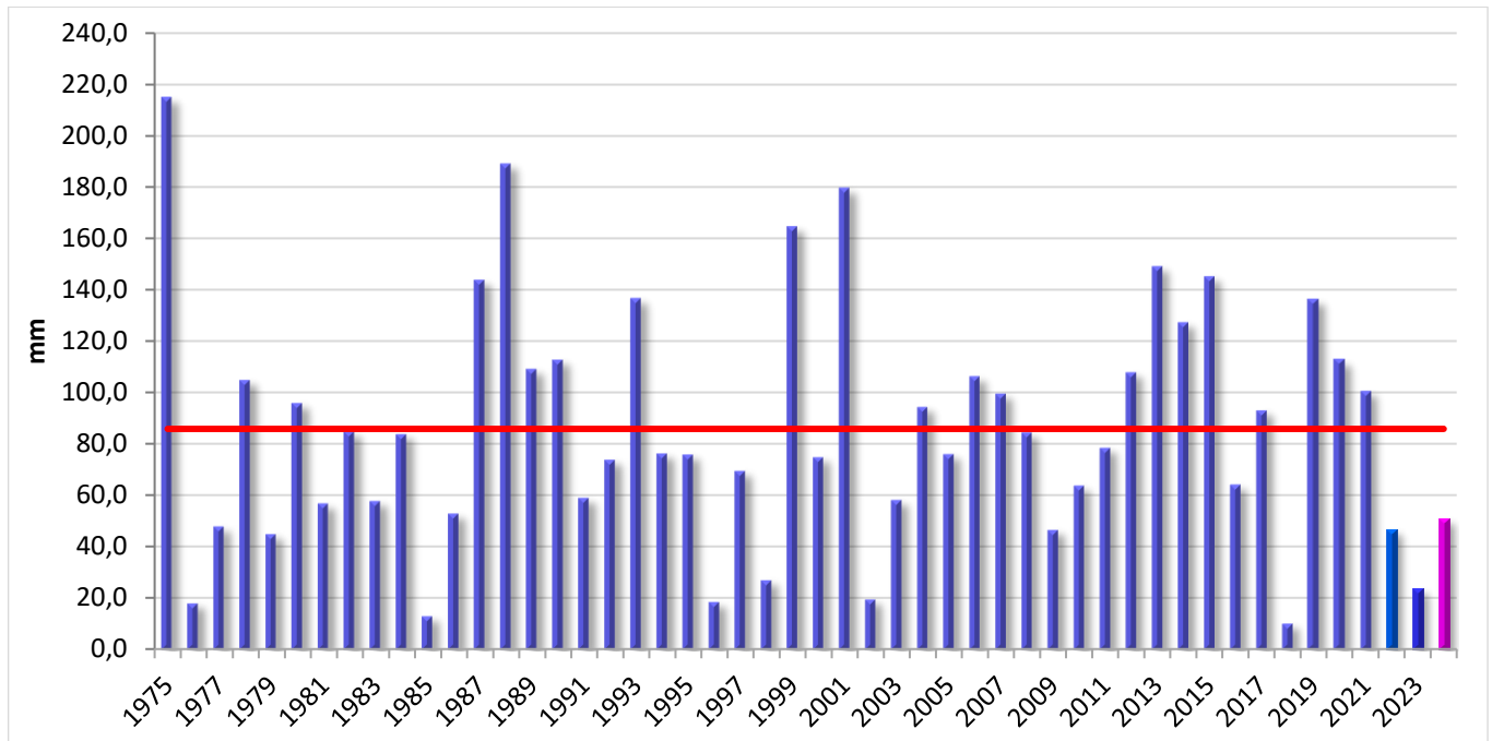
Gráfico 1: Promedio histórico 85.8 mm (línea roja).
