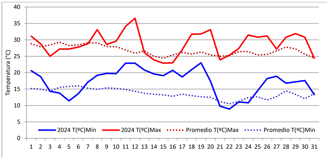
Gráfico 3. Temperaturas Máximas y Mínimas ocurridas durante el mes de Marzo. Las líneas de puntos representan el promedio histórico.
